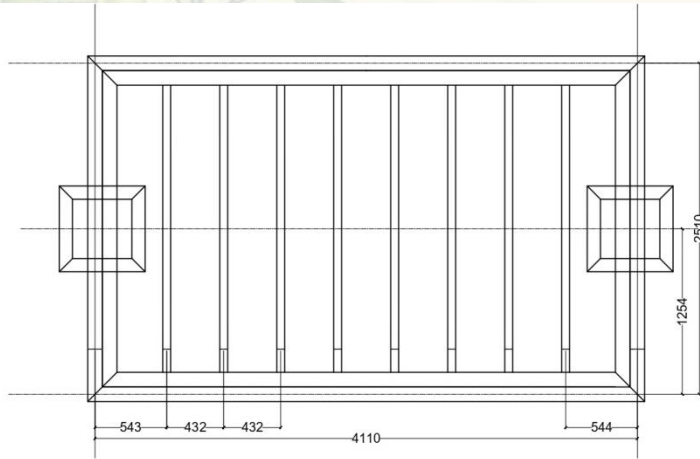
Y-Trellis-Plan
